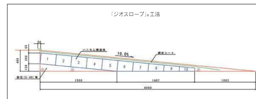
標準断面図 (H=40cm、勾配10%の段差の場合)
