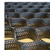
ハニカム構造体(高密度ポリエチレン)
